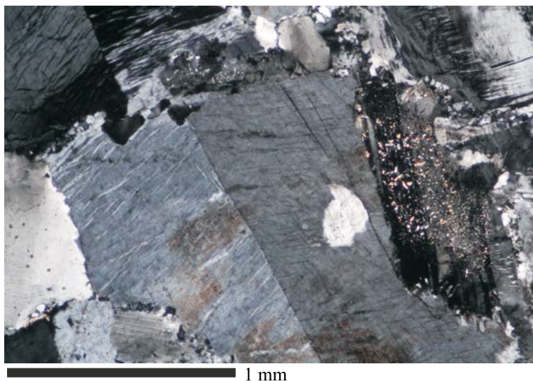
Rys. 1. Mikropertyt mikroklinowy z plamiciem rozłożonym pigmentem, zserycytzowany plagioklaz, kwarc. PX
